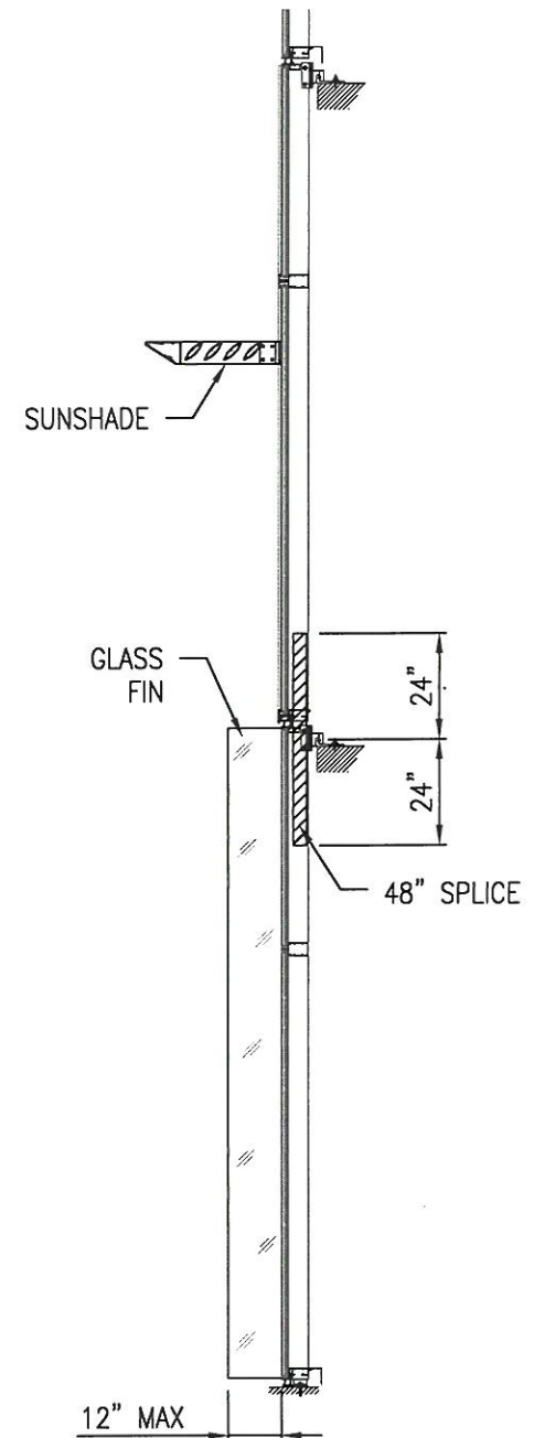
B-B SECTION Scale: 1/4" = 1'-0"
