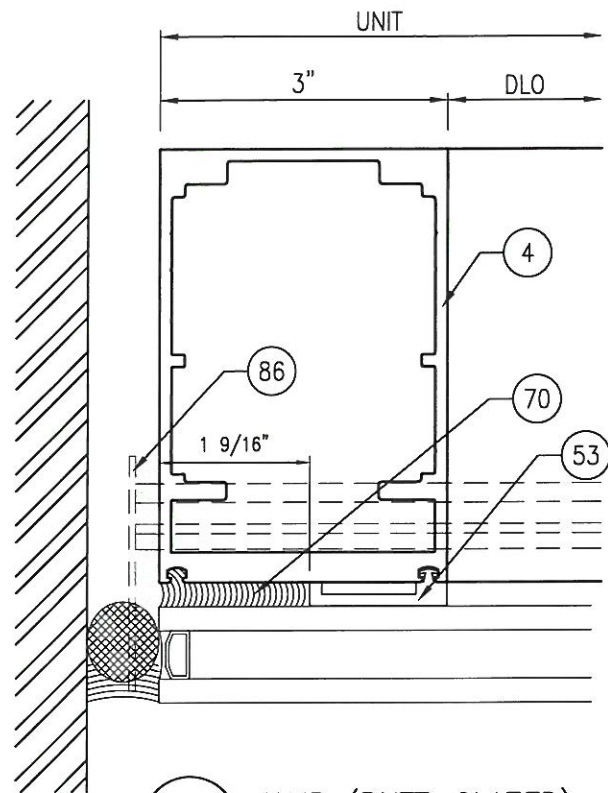
3A JAMB (BUTT-GLAZED) Scale: 6" = 1'-0"
