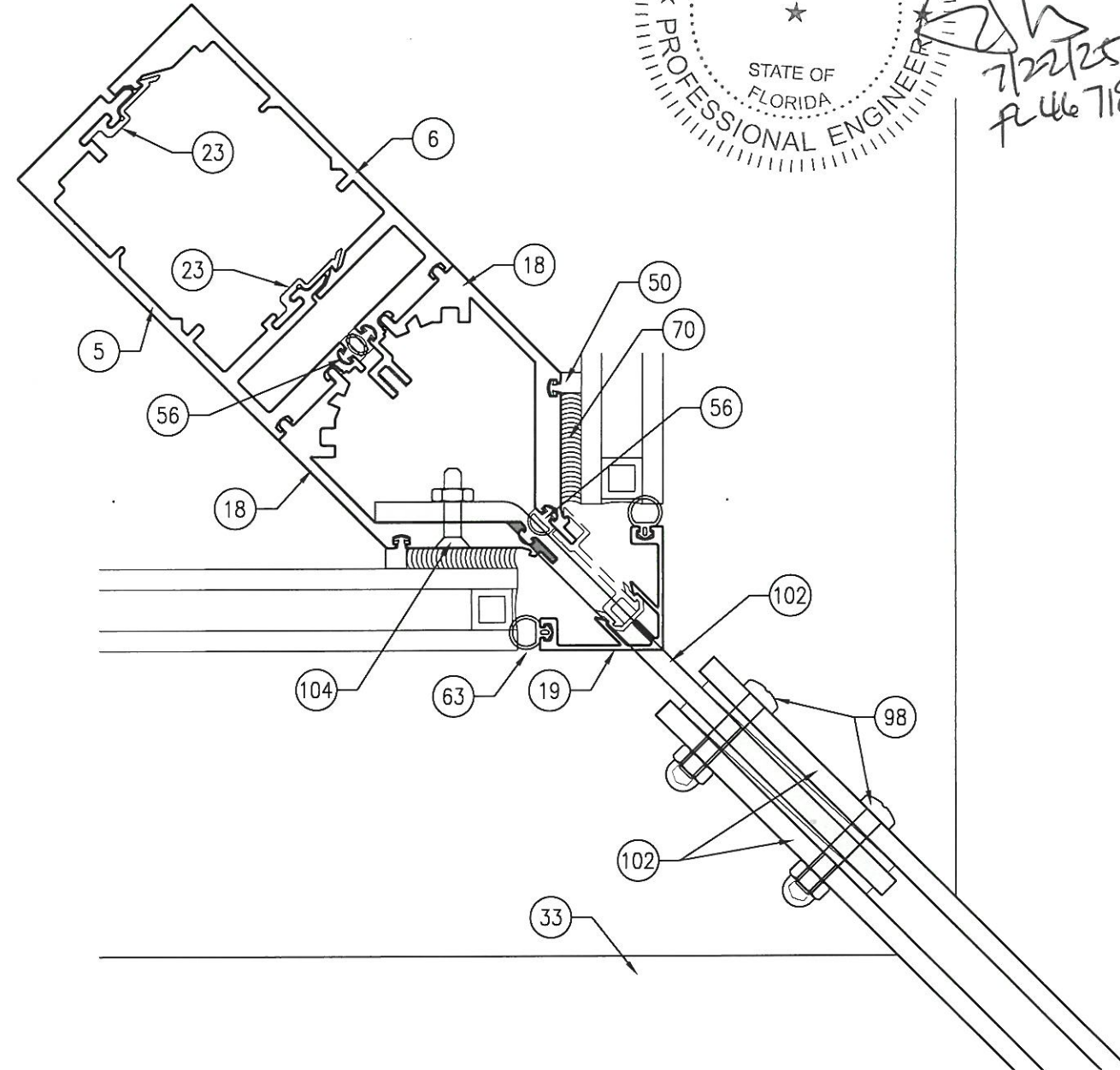
22 SUNSHADE CLIP CORNER Scale: 1:1
