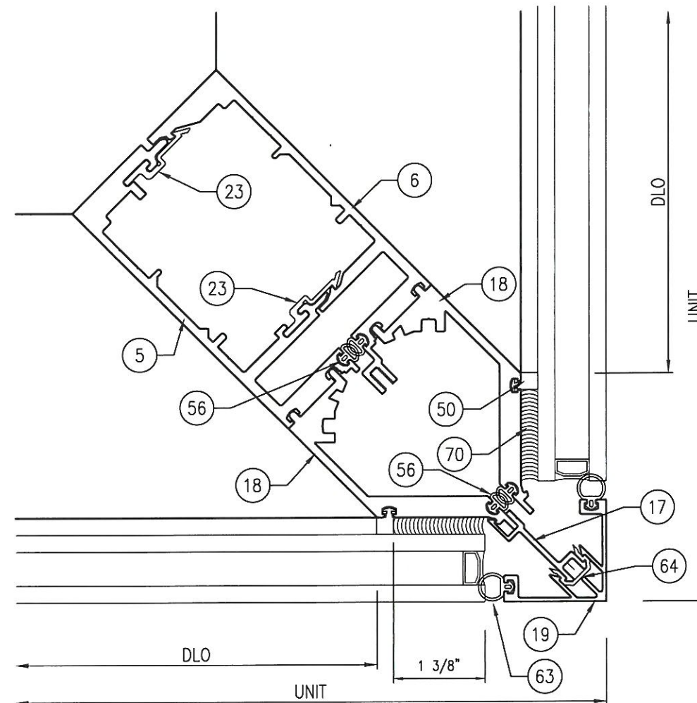
5 90° CORNER Scale: 6" = 1'-0"
