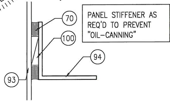
17 PANEL STIFFENER Scale: 6" = 1'-0"
